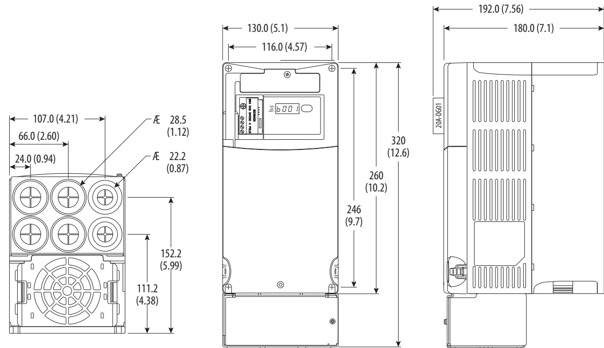
Frame C - 22-JBAC
